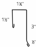
2. Rake Trim
